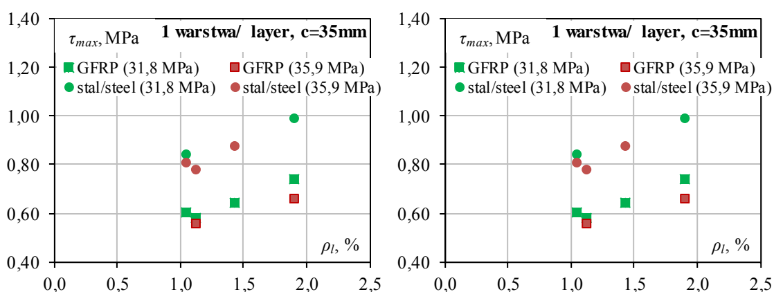
Rys. 4.6. Porównanie maksymalnych naprężeń ścinających w elementach zbrojonych prętami stalowymi oraz GFRP Fig. 4.6. Comparison of maximum shear stresses in steel and GFRP reinforced beams
