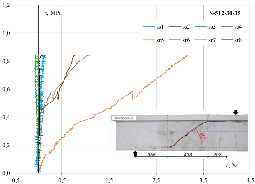
Odkształcenia w strefie ściskanej i rozciąganej – belka S-512-30-35 Concrete strain in compressive and tensile zone – beam S-512-30-35
