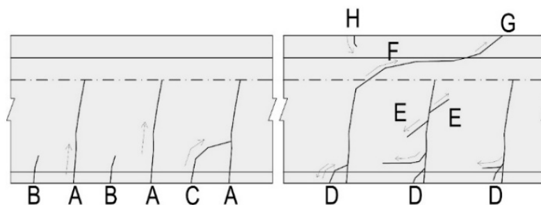
Rys. 3.7. Rodzaje rys w elementach bez zbrojenia poprzecznego Fig. 3.7. Types of cracks in the element without stirrups
