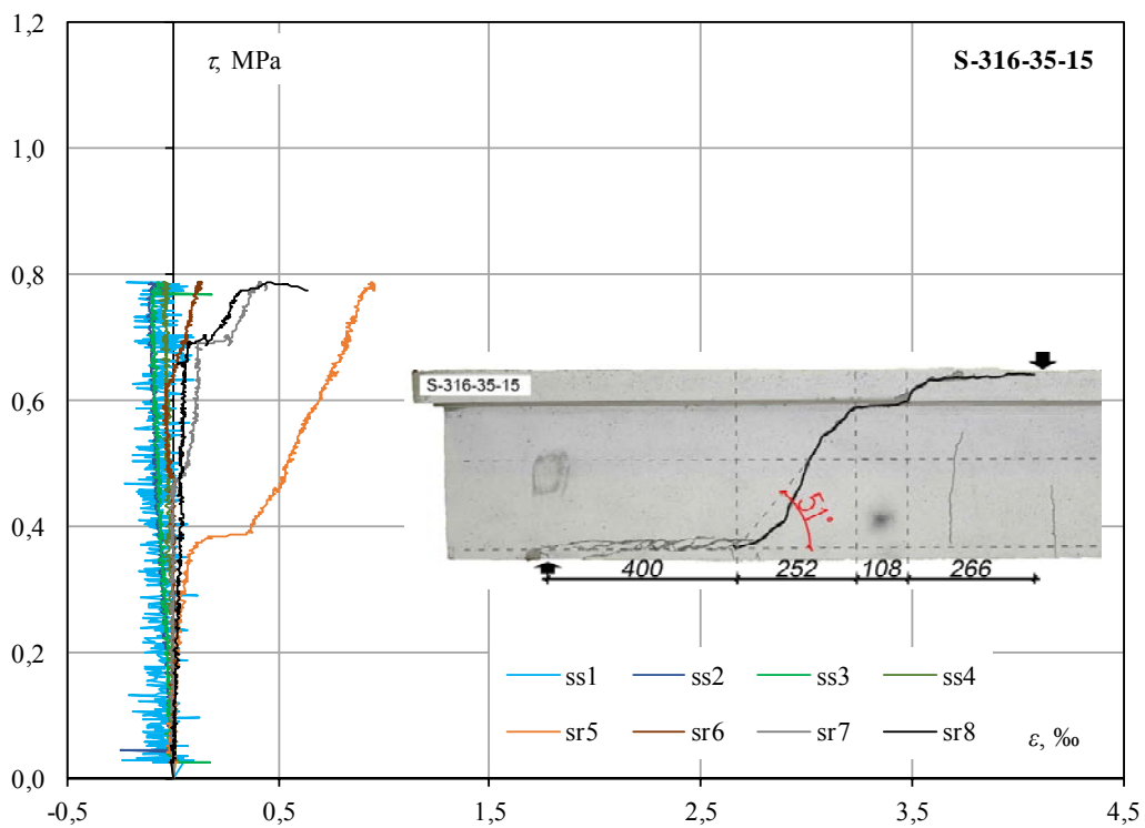
Odształcenia w strefie ściskanej i rozciąganej – belka S-316-35-15 Concrete strain in compressive and tensile zone – beam G-316-35-15
