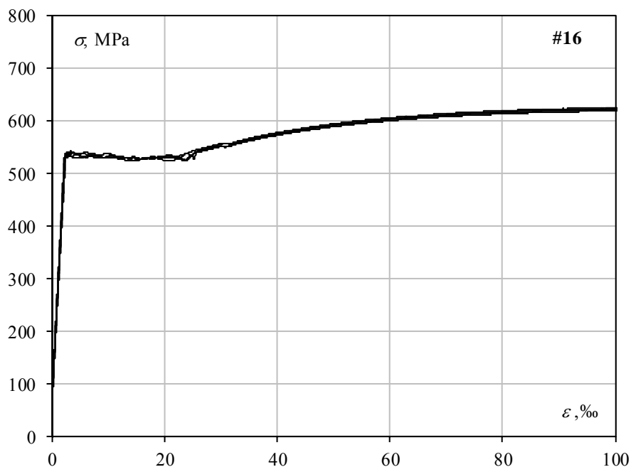
Rys. 3.5. Charakterystyka wytrzymałościowa prętów stalowych o średnicy 16 mm
