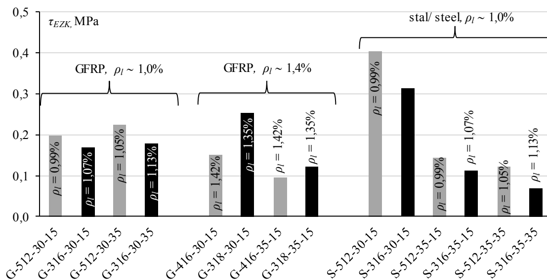
Rys. 4.15. Wpływ liczby prętów i ich średnicy na udział efektu ząbienia kruszywa na niszczące naprężenia ścinające
