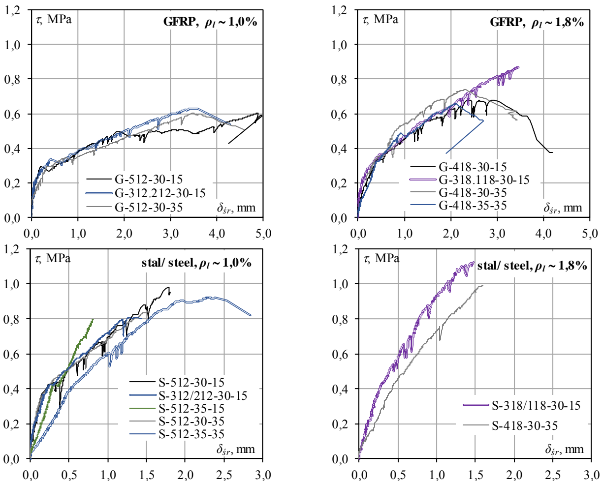
Rys. 4.21. Zależność średniego ugięcia od naprężeń ścinających w elementach z jedną oraz dwiema warstwami zbrojenia Fig. 4.21. Relationship of average deflection vs. shear stresses in elements with one and two reinforcement layers
