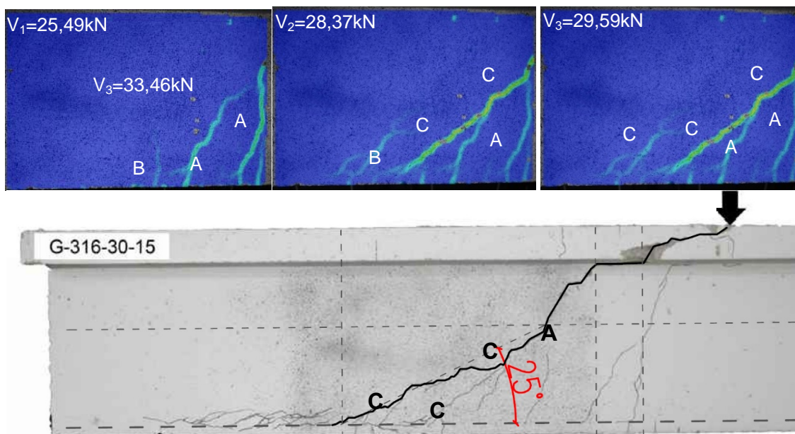
Rys. 3.15. Przykład zniszczenia poprzez połączenie rysy typu „A” i trzech rys typu „C” Fig. 3.15. Failure resulted by connection of cracks “A” and “C” type
