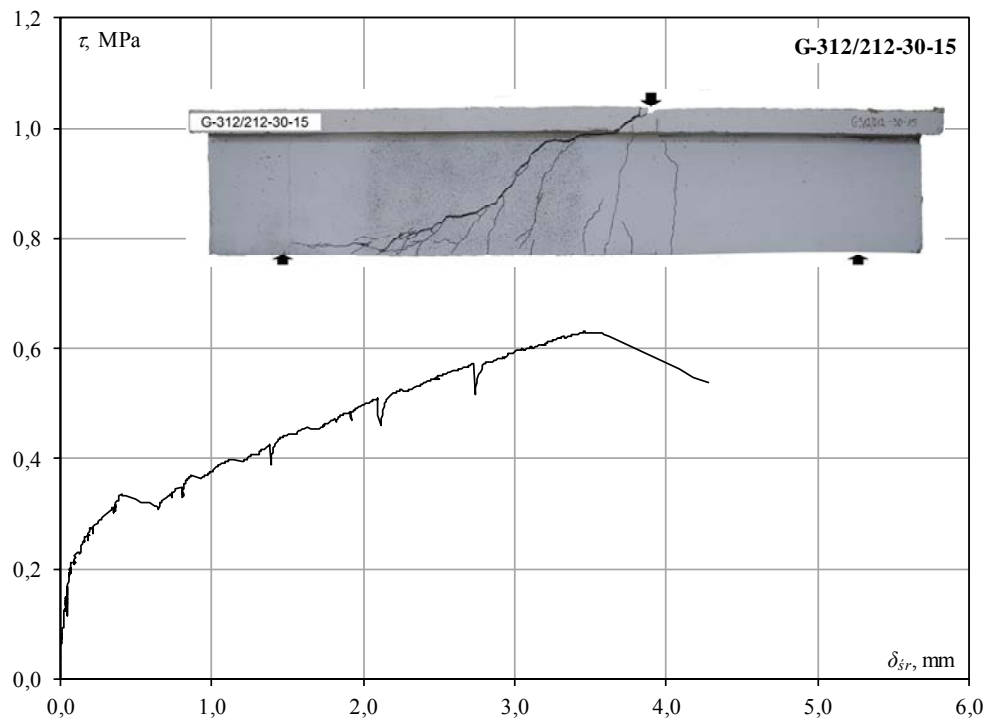
Zależność \tau - \delta_{sr} dla belki G-312/212-30-15 Relationship \tau - \delta_{sr} for beam G-312/212-30-15
