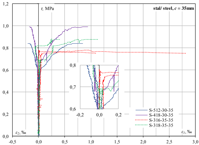
Rys. 3.32. Zależność odkształceń głównych od naprężeń ścinających w badanych belkach ze zbrojenie stalowym, c = 35 \text{ mm}
