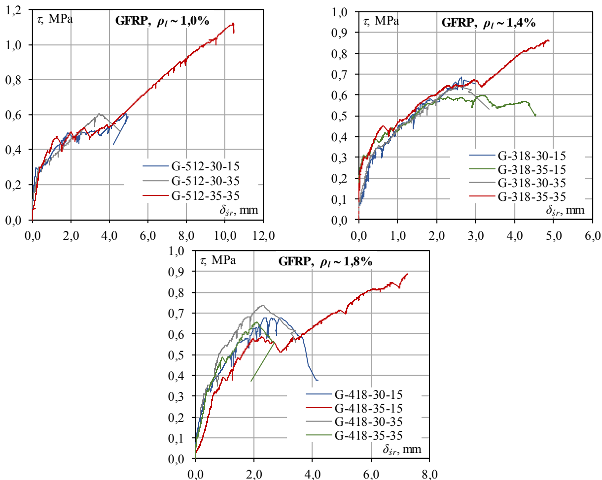
Rys. 4.29. Porównanie zależności naprężenie ścinające – średnie ugięcie w odpowiadających elementach I i II serii, które zniszczyły się na ścinanie i przez utratę przyczepności zbrojenia do betonu
