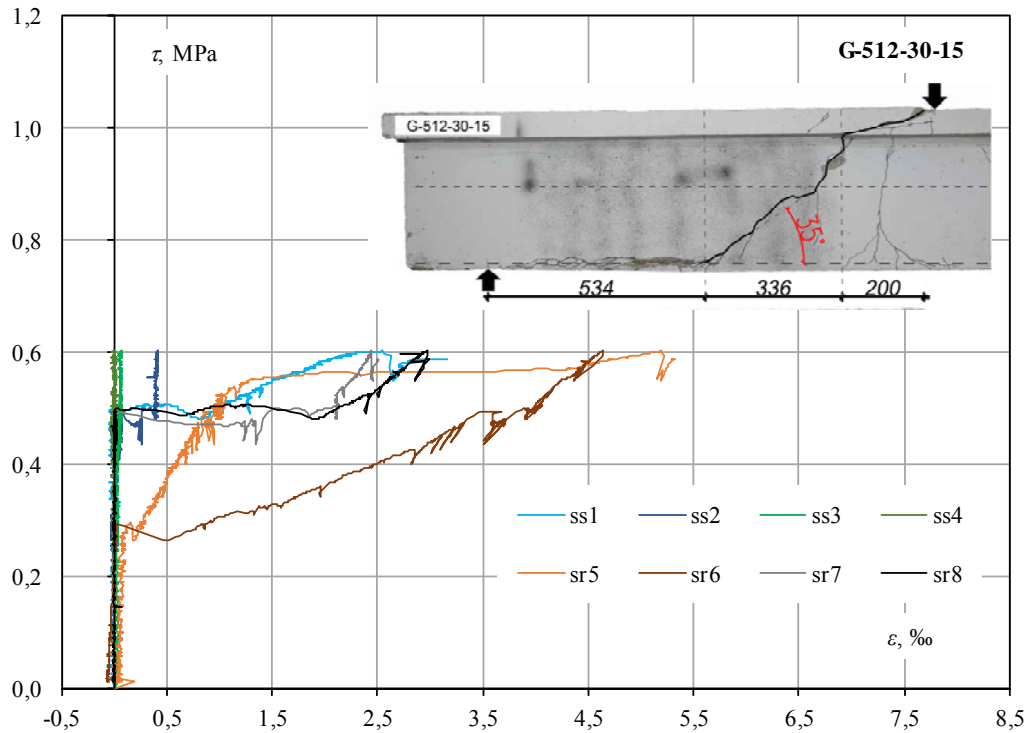
Odkształcenia w strefie ściskanej i rozciąganej – belka G-512-30-15 Concrete strain in compressive and tensile zone – beam G-512-30-15
