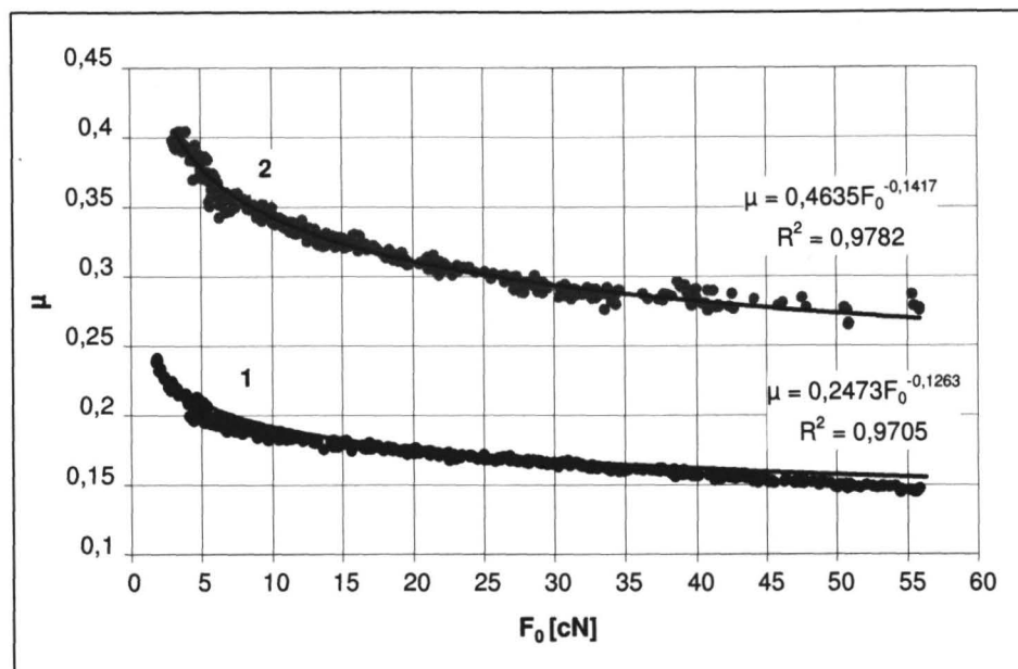
Rys. 3. Wartości umownego współczynnika tarcia \mu w funkcji napięć wstępnych F_0 dla przędzy bawełnianej 20 tex 1 – dla pary ciernych igła – nitka, 2 – dla pary ciernych płaszczka – nitka
