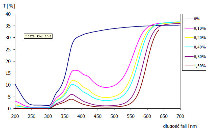
Rys. 13. Transmitancja wybarwionych tkanin z PET w obszarze UV/VIS
